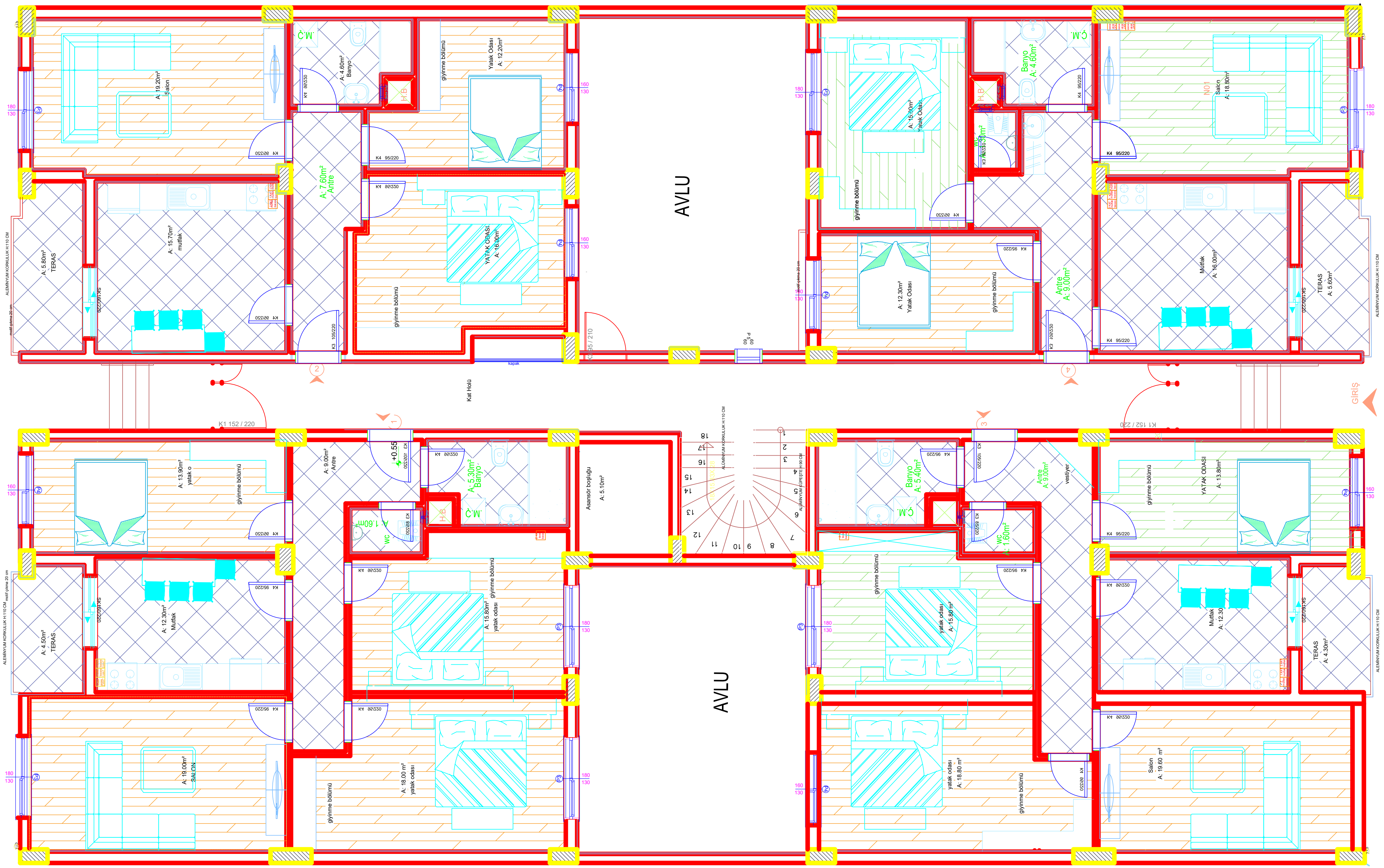
ZEMİN KAT PLANI
